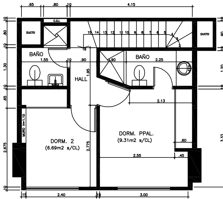
2º PISO DEPTO. DUPLEX DD.1
