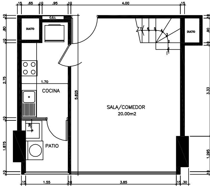
1º PISO DEPTO. DUPLEX DD.1
